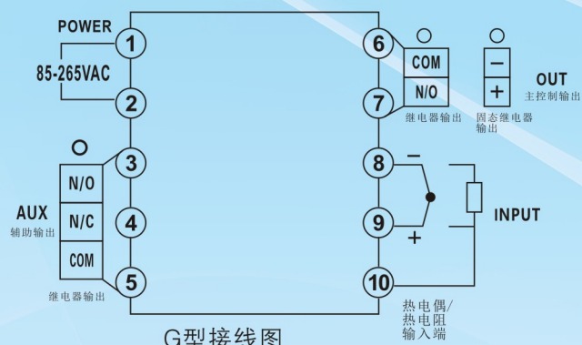
G型接线图
